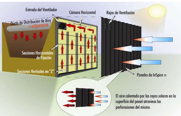
Cómo InSpire™ calienta el aire
